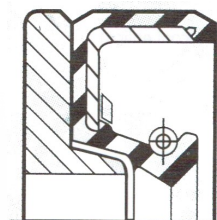
Com anel de apoio Figura 6
