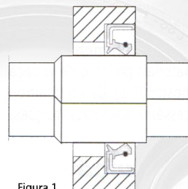
Figura 1 O retentor está montado na parte fixa da máquina com o lábio carregado pela mola em contato com o eixo rotatório.
