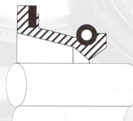
Figura 2 Deve haver uma película fina de óleo entre o lábio e eixo, para reduzir ao mínimo o calor gerado
